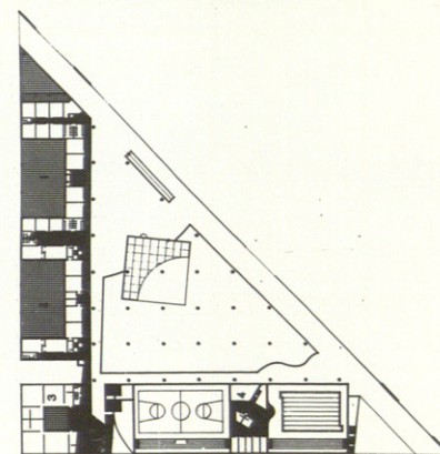
planta +683,50
