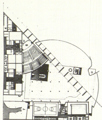
planta +674
